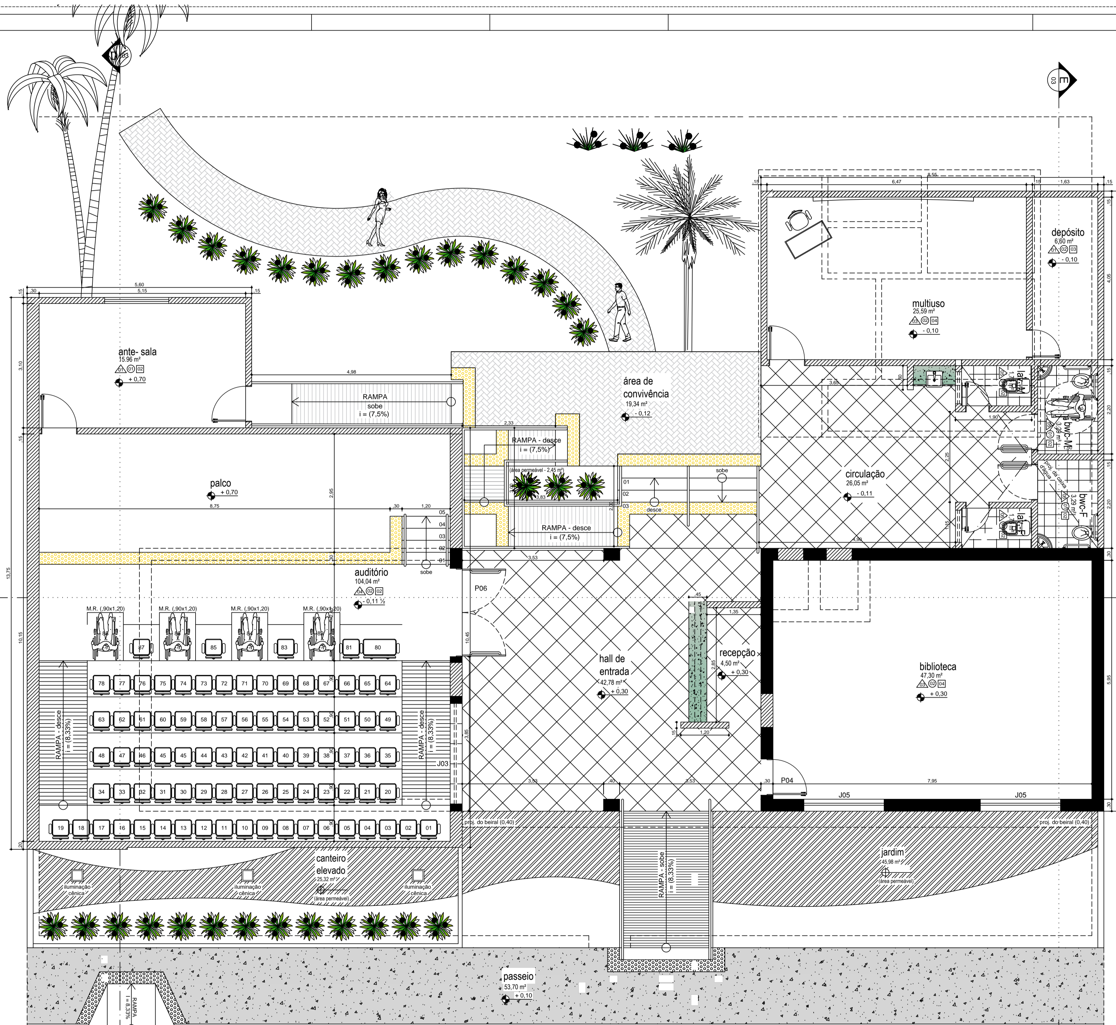
PLANTA BAIXA - TÉRREO ESC: 1:50 ÁREA DE CONSTR. 318,79 m 2
